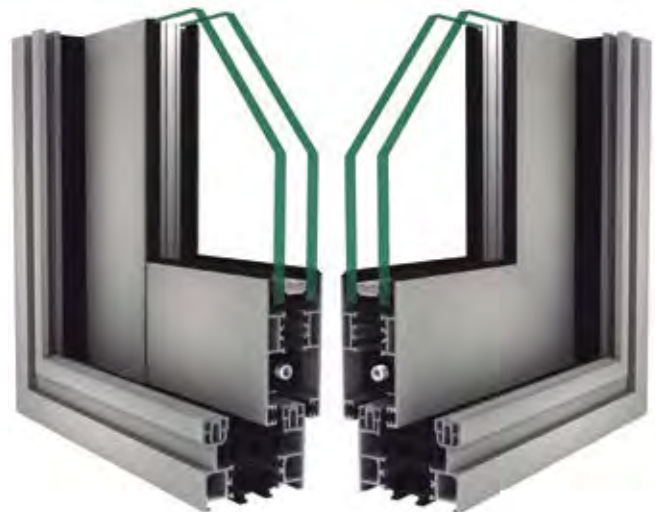
C32 RPT Serie 3600 (Opción Testa y Perimetral)
