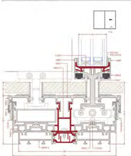
Ventana 1 Hoja - Fijo - Detalle Interior
