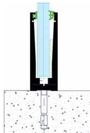
Sobre forjado alineado al exterior
